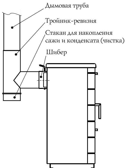
Рисунок 3. Схема присоединения печи к дымоходу.
